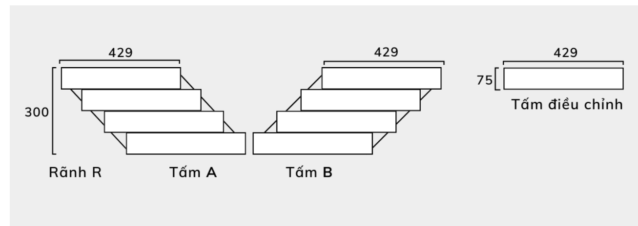
Bản vẽ bề mặt (đơn vị mm)
