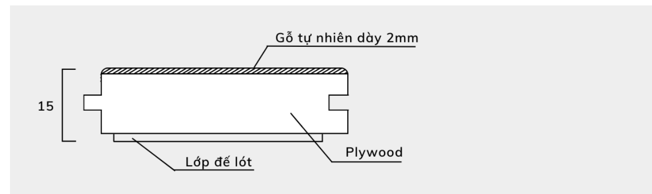
Bản vẽ bề mặt (đơn vị mm)
