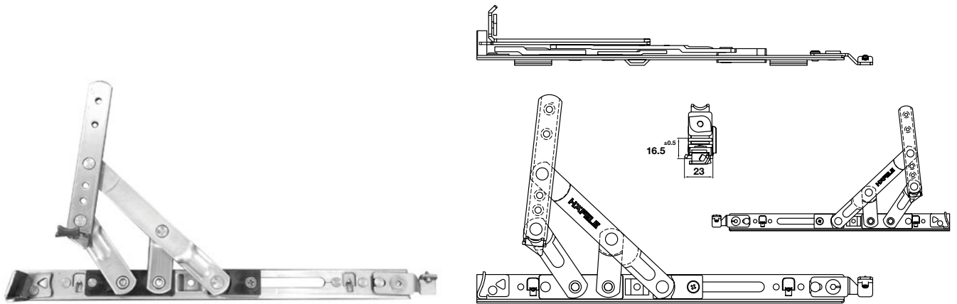
Friction stay / Bản lề chữ A
