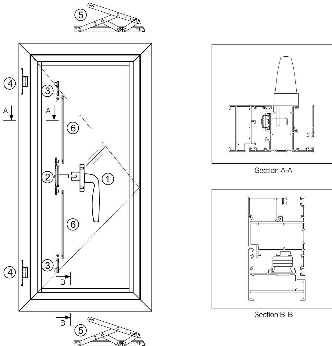
Typical planning for single side hung window Phương án điển hình cho cửa sổ mở xoay 1 cánh
