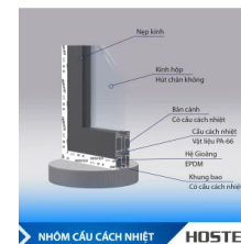
Nhôm cầu cách nhiệt HOSTEN
