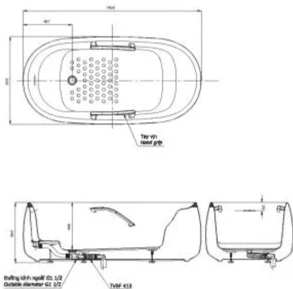
Ảnh 2D của bồn tắm nằm rời Galato PJY1744HPWENMW_TVBF412
